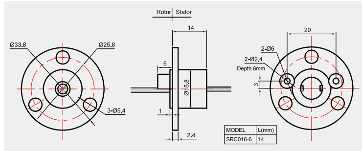
外形尺寸 OUTLINE DIMENSION 单位(UNIT) mm
