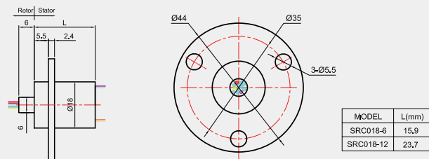
外形尺寸 OUTLINE DIMENSION 单位(UNIT) mm
